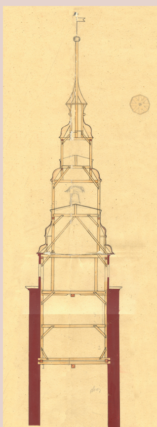
Plánová dokumentace z roku 1865 zachycující v řezu renesanční konstrukci krovu a zdiva Hlášky. Státní okresní archiv Opava
