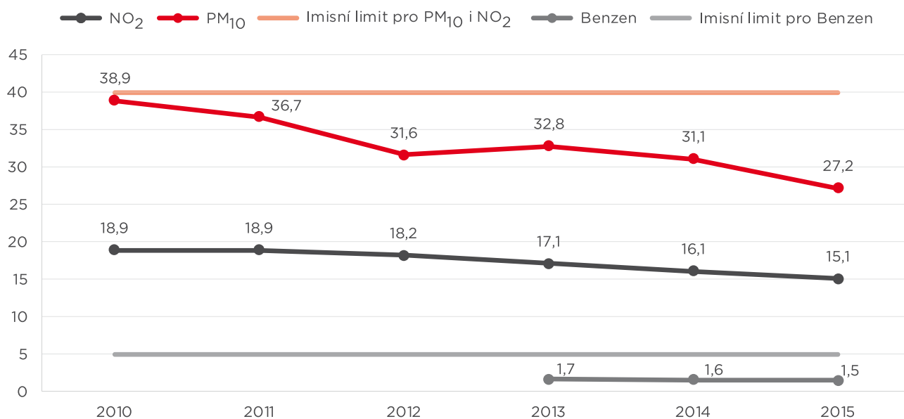
GRAF | Průměrné roční koncentrace vybraných znečišťujících látek a jejich roční imisní limity v letech 2010–2015 na AIMS 1186 Opava-Kateřinky | Zdroj: ČHMÚ
