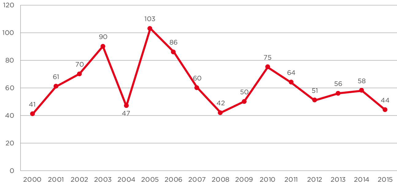
GRAF | Počet překročení 24hodinového imisního limitu ( 50 \mu\text{g}/\text{m}^3 ) pro \text{PM}_{10} v letech 2000–2015 na AIMS 1186 Opava-Kateřinky | Zdroj: ČHMÚ
